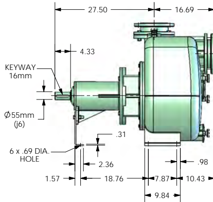
6SJ16 Flange
