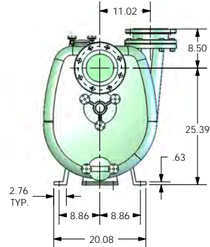
6SJ16 Flange
